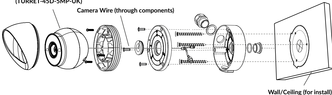
IP Camera (TURRET-45D-5MP-UK)
